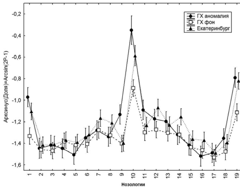
Рис. 2. Средняя частота регистрации заболеваний по отдельным нозологиям* на геохимически контрастных территориях
