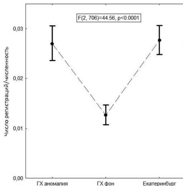
Рис. 1. Средняя частота регистрации заболеваний (все нозологии) по отношению к численности населения исследуемого района на геохимически контрастных территориях. Возраст (дети: от 0 до 14 лет, подростки: от 14 до 17 лет, взрослые: старше 18 лет) использован как ковариата. ГХ аномалия – естественная геохимическая аномалия (пос. Уралец), ГХ фон – геохимически фоновый участок (Шалинский район).
