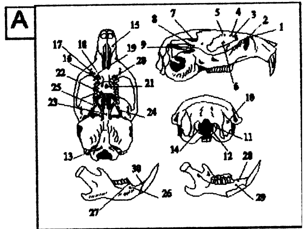
Рис.1. Фенетический анализ импактной и контрольных популяций модельного вида-радиофора в Каменском районе Свердловской области в зоне ВУРС.
