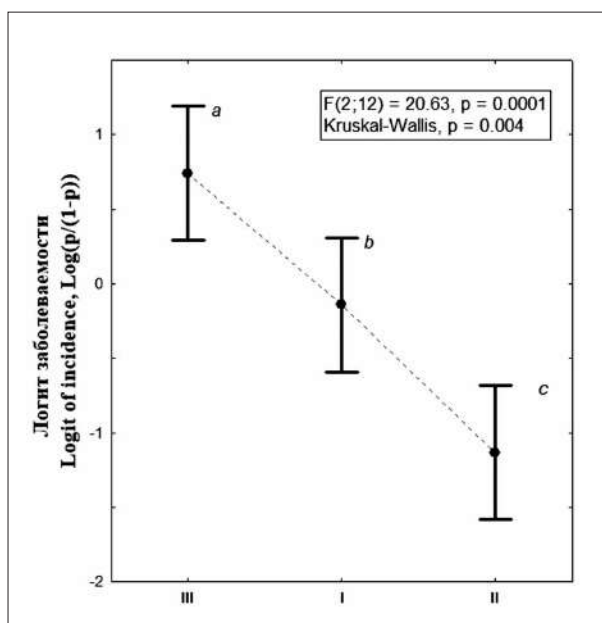
Рис. 1. Результаты ANOVA для логарифмов шансов (логиты, LogOdds) заболевания (в год): I – Екатеринбург; II – биогеохимический фон; III – биогеохимическая провинция. Не содержащие одинаковых символов оценки (a, b, c) статистически значимо различаются, p < 0,05
