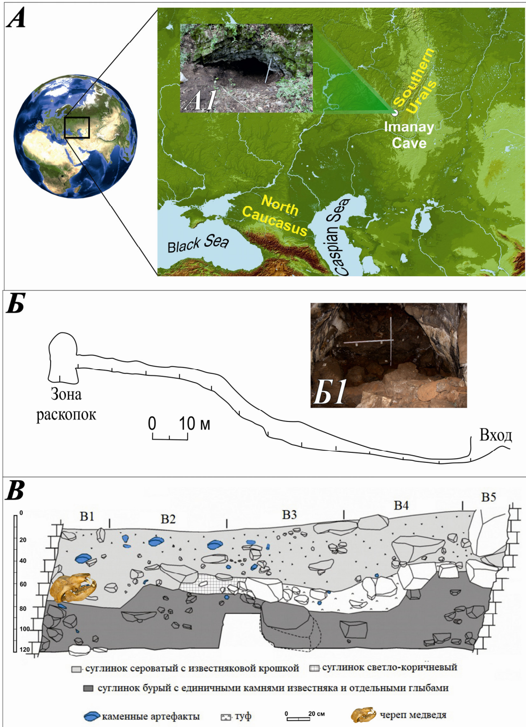
Рис. 1. Географическое положение, морфология и стратиграфия рыхлых отложений пещеры Иманай: А — география и внешний вид входа в пещеру (А1); Б — план-схема пещеры и вид на раскоп (Б1); В — стратиграфия рыхлых отложений пещеры и место находки черепа медведя.
