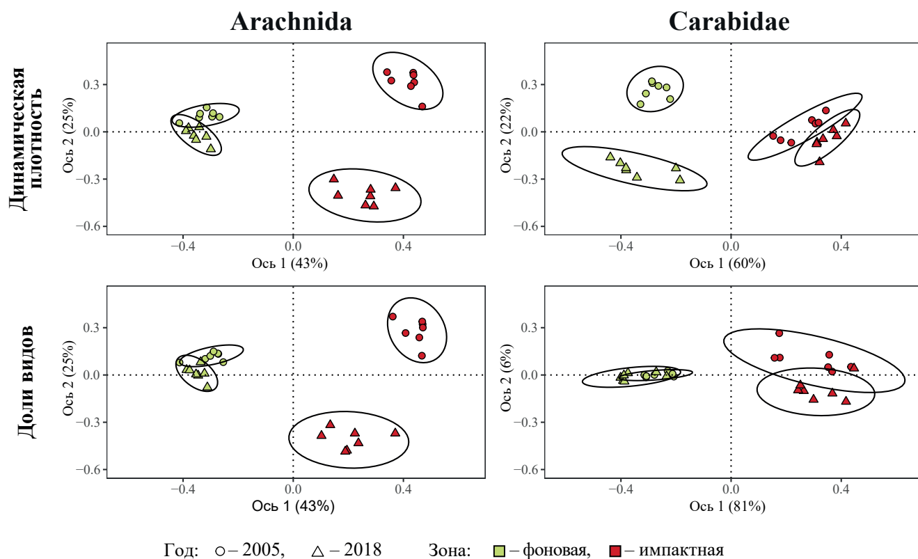
Рис. 2. Ординация (на основе расстояния Брея-Кертиса) комплексов паукообразных (Arachnida) и жужелиц (Carabidae) сравниваемых участков и периодов по абсолютному (динамическая плотность) и относительному (доли видов) обилию. Показаны 95%-ные эллипсы, в скобках – доля объясняемой дисперсии, %.
