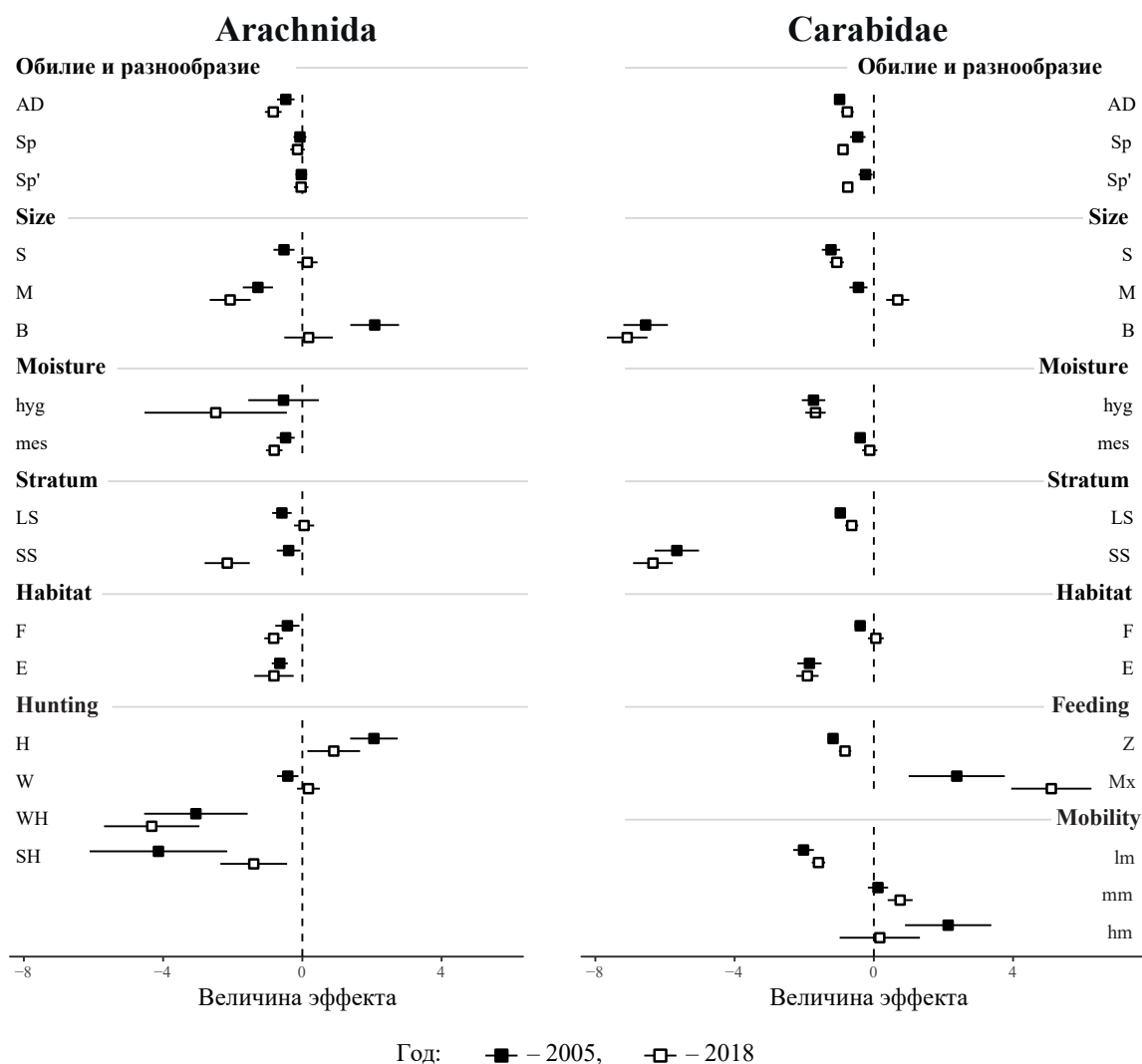
Рис. 1. Величина эффекта и ее 95%-ный доверительный интервал для сравниваемых периодов (2005 г. и 2018 г.). Обозначения экологических групп паукообразных (Arachnida) и жулици (Carabidae) указаны в табл. 1. Параметры разнообразия и обилия: AD – динамическая плотность, Sp – наблюдаемое число видов, Sp' – интерполированное к 100 особям число видов.
