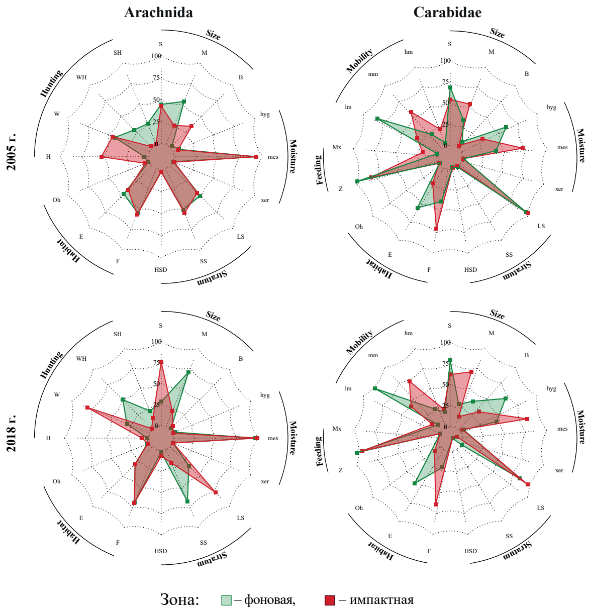
Рис. 3. Экологические профили (доли групп, %) комплексов паукообразных (Arachnida) и жуужелиц (Carabidae) сравнимых участков и периодов. Обозначения свойств и экологических групп указаны в табл. 1.
