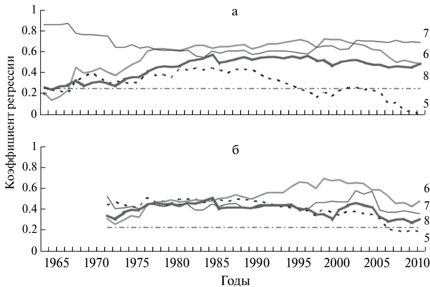
Рис. 8. Климатический отклик MXD сосны на температуру летних месяцев на основе 30-летнего скользящего осреднения.
