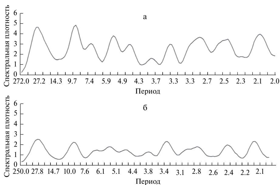
Рис. 10. Спектральная плотность реконструированных рядов. а – Усинск, б – Печора.
