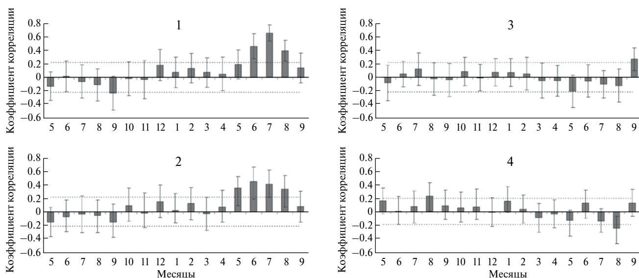
Рис. 7. Связь между MXD сосны и средней месячной температурой (1,2) и суммой осадков (3,4) за период с мая предшествующего года по сентябрь текущего на местообитании Усинск (1, 3) и Печора (2, 4). Горизонтальные линии – уровень достоверности p < 0.05 .
