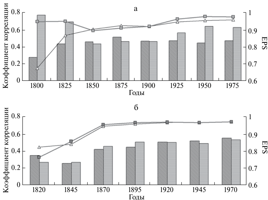
Рис. 5. Коэффициенты EPS (линия) и скользящей средней корреляции между сериями ( r_{\text{bar}} ) (столбики) по ШГК (серым цветом) и MXD (черным цветом). а – Усинск, б – Печора.
