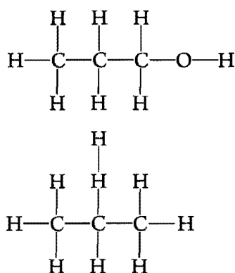
Рис. 11. Два изомера пропилового алкоголя.
