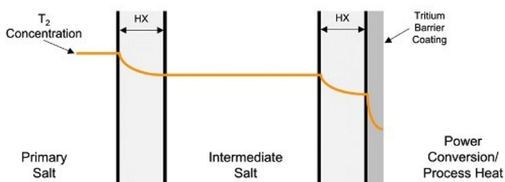
Рис. 1.3. Вариант размещения антритриевого барьера ( http://www.atominfo.ru/newsz02/a0128.htm )
