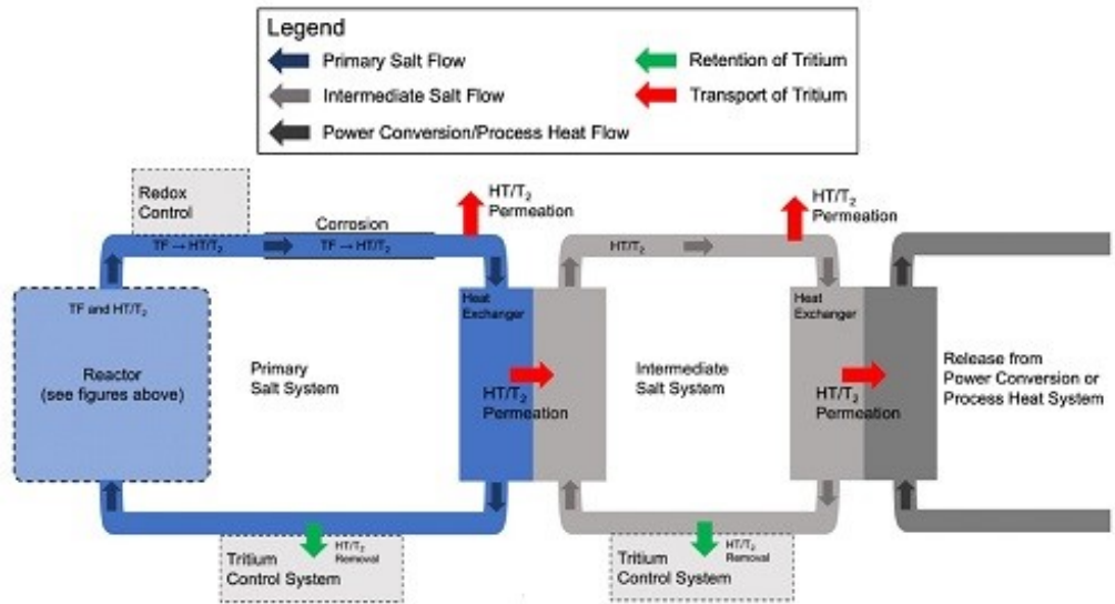
Рис. 1.2. Барьеры в ПВ-FHR, MSR и в контурах ЖСР ( http://www.atominfo.ru/newsz02/a0128.htm )
