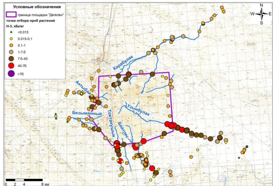
Рис. 4.30. Карты-схемы распределения трития: a — в воздушном бассейне (по данным объёмной активности ^3\text{H} в почвенном воздухе); б — в растительном покрове (по данным удельной активности ^3\text{H} в свободной воде растений) [К вопросу о путях..., 2014]
