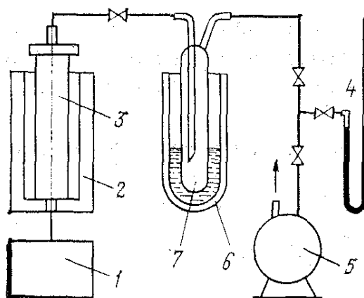
Рис. 1.23. Схема установки для термовакуумной десорбции воды:
