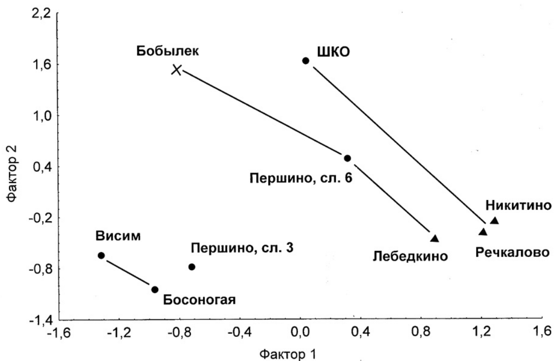
Рис. 3. Расположение выборок в координатах 1 и 2 факторов. Точками обозначены местонахождения предгорий, треугольниками - на равнине, крестиком - на западном склоне Урала. Сплошными линиями соединены близкие по возрасту местонахождения.
