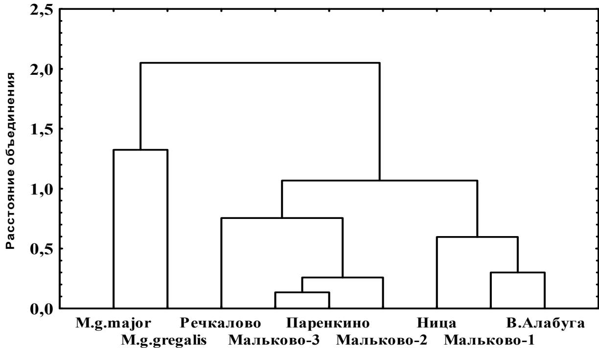
Рис. 7. Сравнение ископаемых и современных выборок узкочерепной полевки методом полной связи (Евклидово расстояние): Возраст местонахождений см. рис. 6. Современные подвиды: M.g. gregalis (Камышлов), M.g. major (п-ов Ямал).
