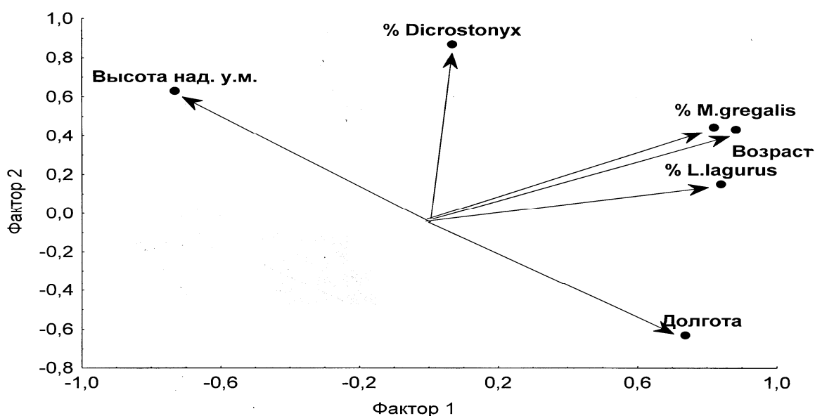
Рис. 2. Расположение признаков в координатах 1 и 2 факторов.
