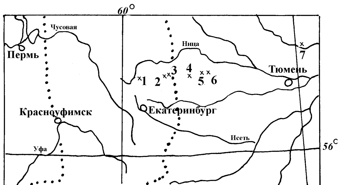
Рис. 1. Карта расположения новых местонахождений четвертичных фаун Зауралья: 1 - ШКО; 2- Першинская пещера; 3 - Босоногая; 4 - Лебедкино; 5 - Речкалово; 6 - Никитино; 7 - Нижняя Тавда. Пунктирная линия - граница Уральских гор.
