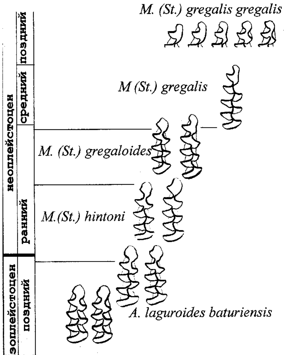
Рис. 5. Схема эволюции линии Allophajomys laguroides baturiensis - ( M. ) Stenocranius gregalis (по М 1 ).
