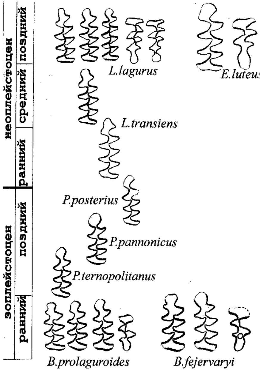
Рис. 4. Схема эволюции рода Borsodia и полевок трибы Lagurini (по М 1 , М 3 ).
