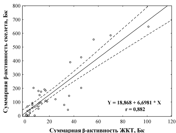
Рис. 1. Зависимость суммарной \beta -активности скелета от \beta -активности желудочно-кишечного тракта (ЖКТ). Пунктирные линии (здесь и на рис. 2, 3) – границы 95%-ного доверительного интервала
