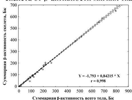
Рис. 3. Зависимость суммарной \beta -активности скелета от \beta -активности всего организма
