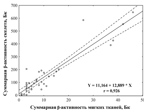
Рис. 2. Зависимость суммарной \beta -активности скелета от \beta -активности мягких тканей
