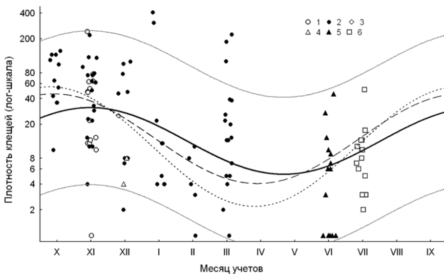
Рис. 2. Динамика плотности (жирная линия — ожидаемое значение E(y) , пунктир — 95% ПИ — предсказываемый интервал) гемазового клеща Macronyssus corethroproctus у зараженных? (Балашов и др. такой термин не используют) особей прудовой ночницы ( n > 0 ).
