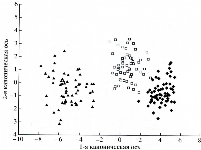
Рис. 3. Распределение экземпляров лесных полевок в пространстве 1 и 2 дискриминантных канонических осей. Темный треугольник – Cl. rufocanus , светлый квадрат – Cl. glareolus , темный ромб – Cl. rutilus .
