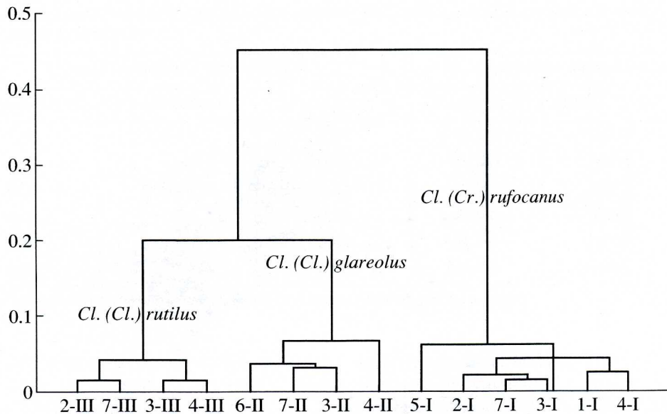
Рис. 2. Классификация выборок полевок рода Clethrionomys по средним значениям длины и ширины жевательной поверхности M^2 (метод UPGMA, евклидово расстояние). I – Cl. rufocanus , II – Cl. glareolus , III – Cl. rutilus . Номера выборок – см. табл. 1.
