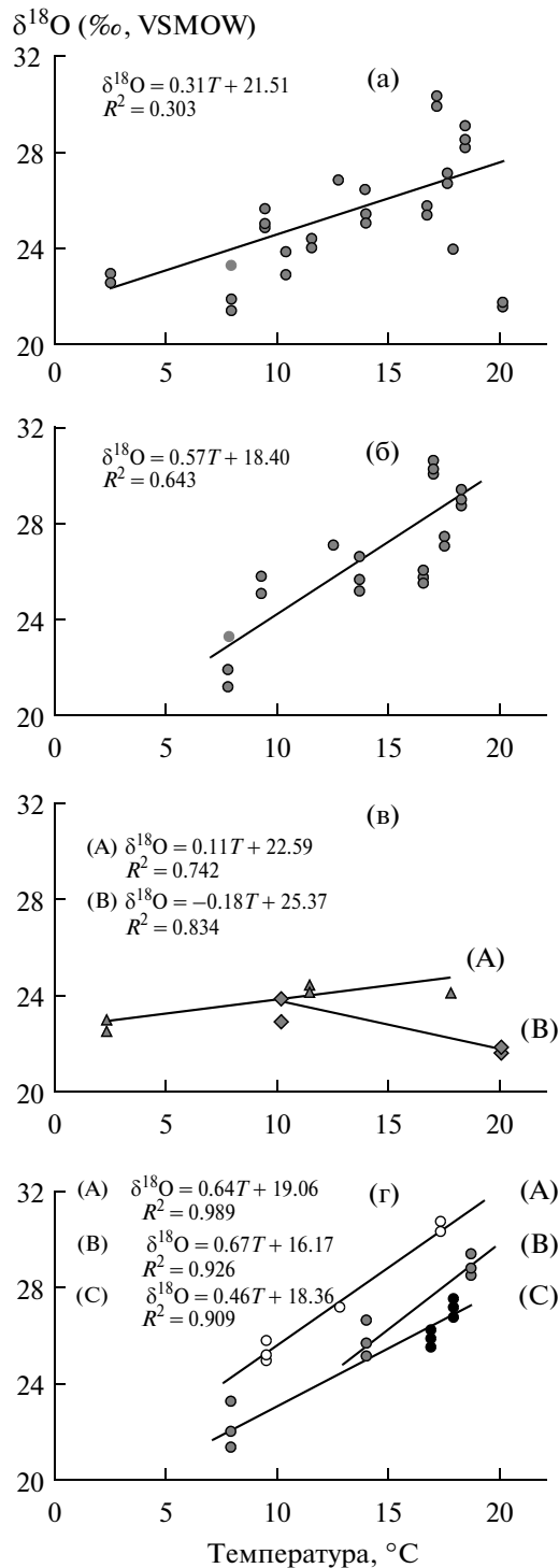
Рис. 2. Изотопный состав кислорода \delta^{18}\text{O} карбонатной группы гидроксилатапта в резцах исследуемых грызунов относительно температуры окружающего воздуха.
