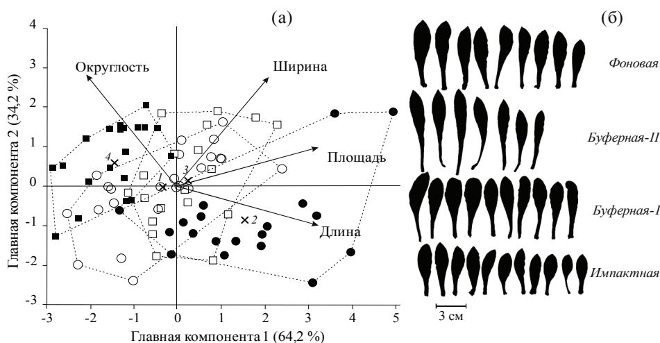
Рис. 1. Результаты анализа формы и размера листьев L.flos-cuculi из разных зон загрязнения (фоновой ○, буферной-II ●, буферной-I □, импактной ■) с помощью метода главных компонент (а), крестиками указаны центры популяций (фоновой – 1, буферной-II – 2, буферной-I – 3, импактной – 4). Типичные листья в разных популяциях (б). Показаны листья особей, наиболее близких к центрам популяций
